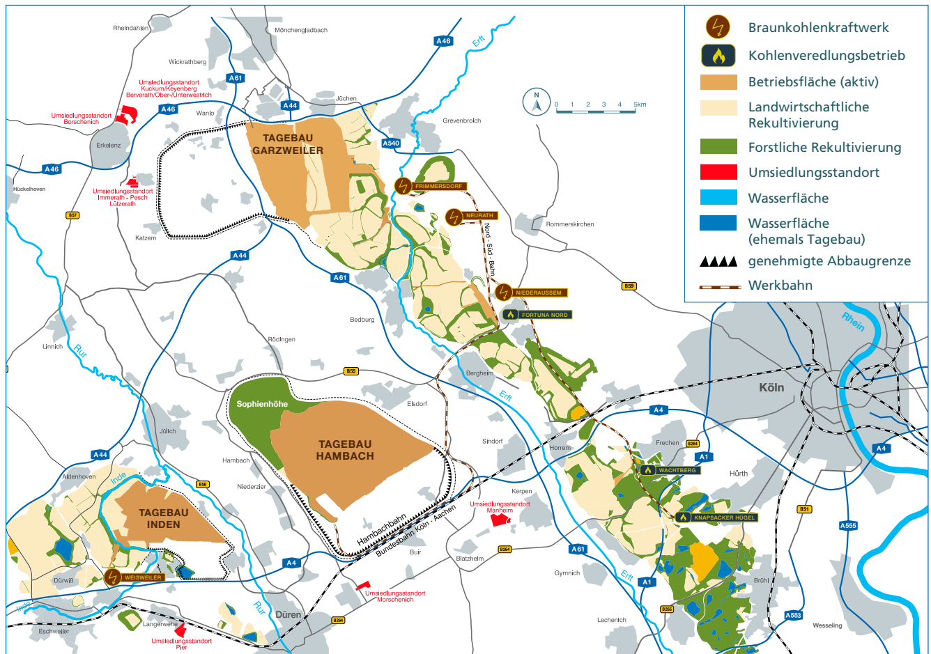
Abbildung 18: Rheinisches Revier
