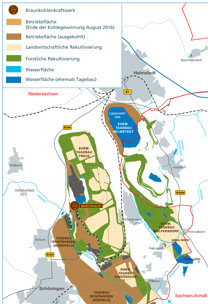
Abbildung 22: Helmstedter Revier
