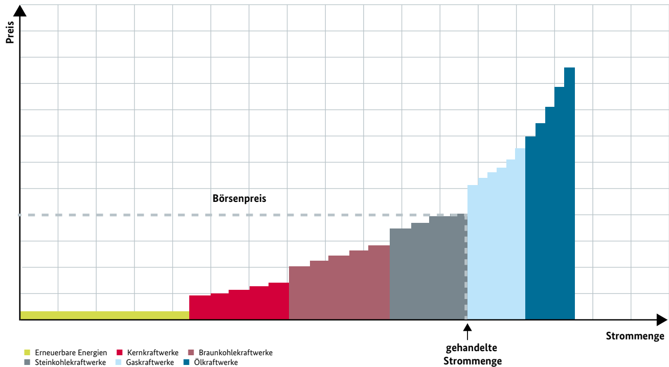
Abbildung 6: Merit Order
